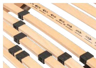
SISTEMA REGOLATORI DI RIGIDITÀ SU DOPPIA DOGA SOVRAPPOSTA
